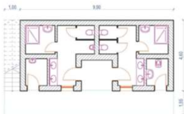
Tloris nadstropja
