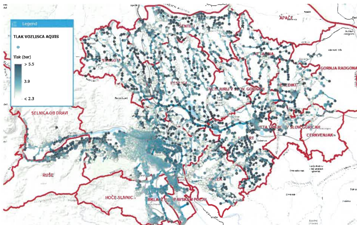
Slika 1: Tlačne razmere v omrežju
